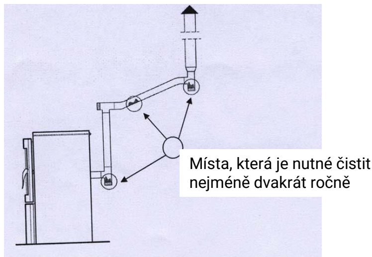
Obrázek 15. Místa, která je nutné čistit nejméně dvakrát ročně
