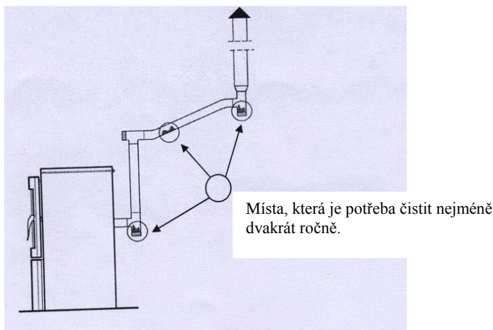
Obrázek 18. Místa, která je potřeba čistit nejméně dvakrát ročně
