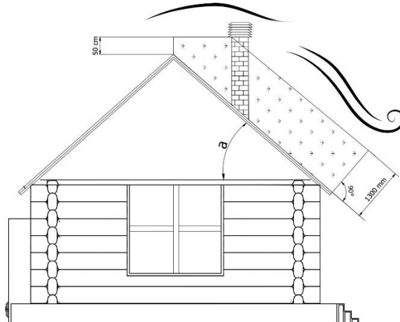
Je zakázáno používat komínové trubky s vnitřní pravouhlou částí, které se liší od plánu. Účinnost pouhých 40%
